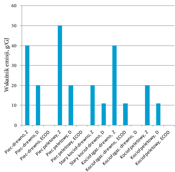
Rys. 18. Emisja zanieczyszczeń ze spalania drewna i pellet w różnych urządzeniach grzewczych Z – stara technika, D – nowa technika, ECOD – wymogi dyrektywy ErP
